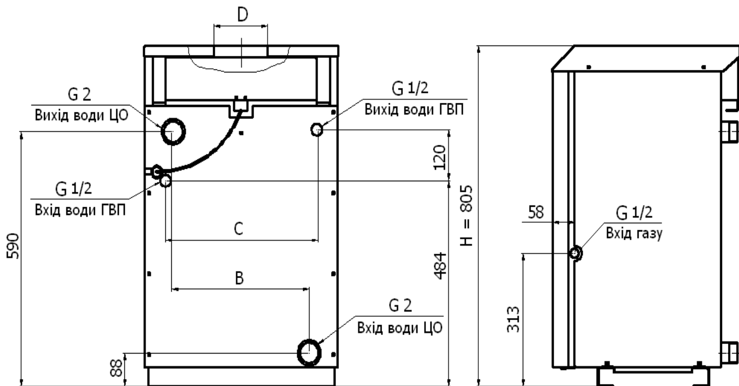
Рисунок 2. Приєднувальні розміри котла опалювального сталевого АОГВ-25КСС/КСВС та АОГВ-30КСС/КСВС( вид ззаду)
