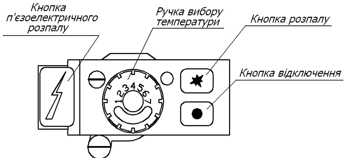
Рисунок 3. Елементи управління газового клапану 710 MINISIT.
