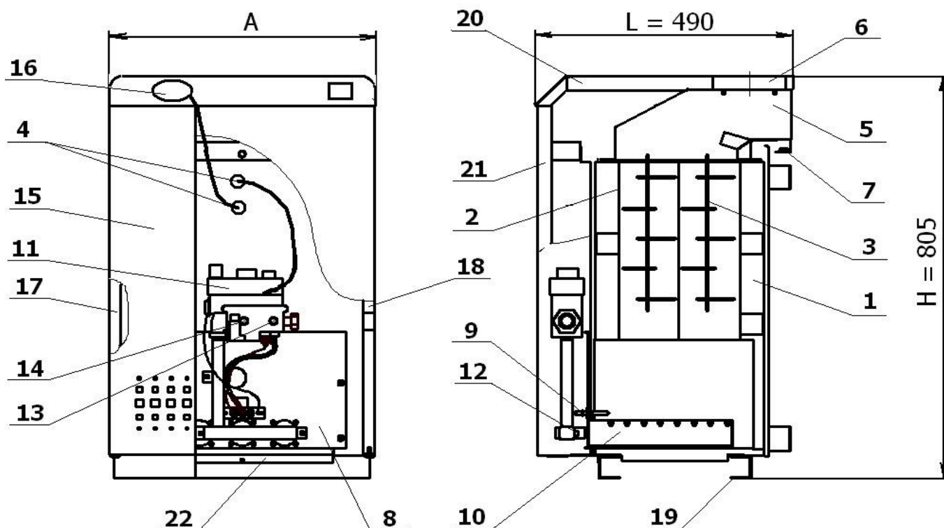
Рисунок 1. Котел опалювальний сталевий АОГВ-25КСС/КСВС та АОГВ-30КСС/КСВС.
